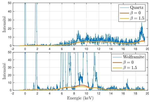
FIGURE 2 : Exemples de lignes de base obtenues sur deux pixels de l'image hyperspectrale XRF. Un spectre de quartz (en haut) et un spectre de wolframite (en bas)
